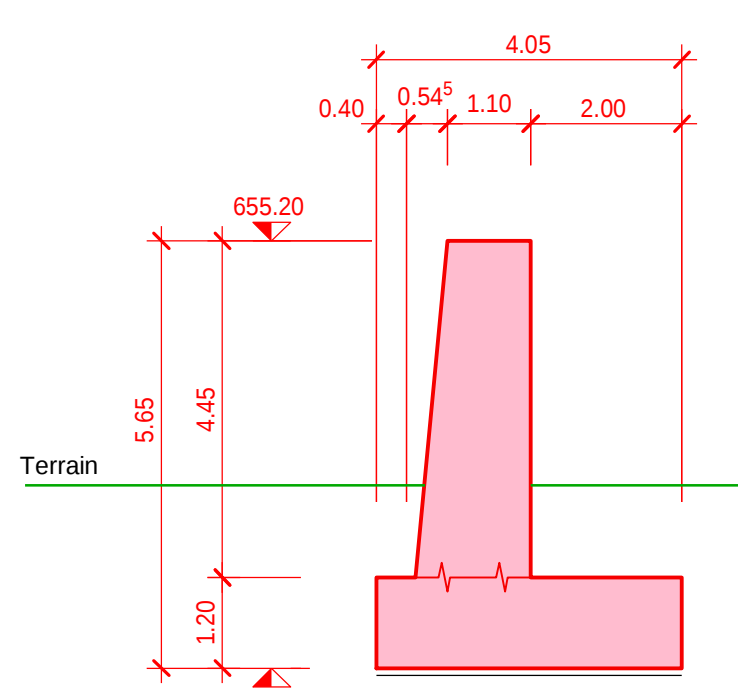
Schnitt E 1:100
