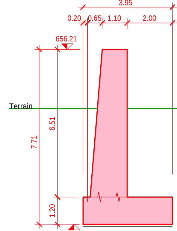
Schnitt F 1:100
