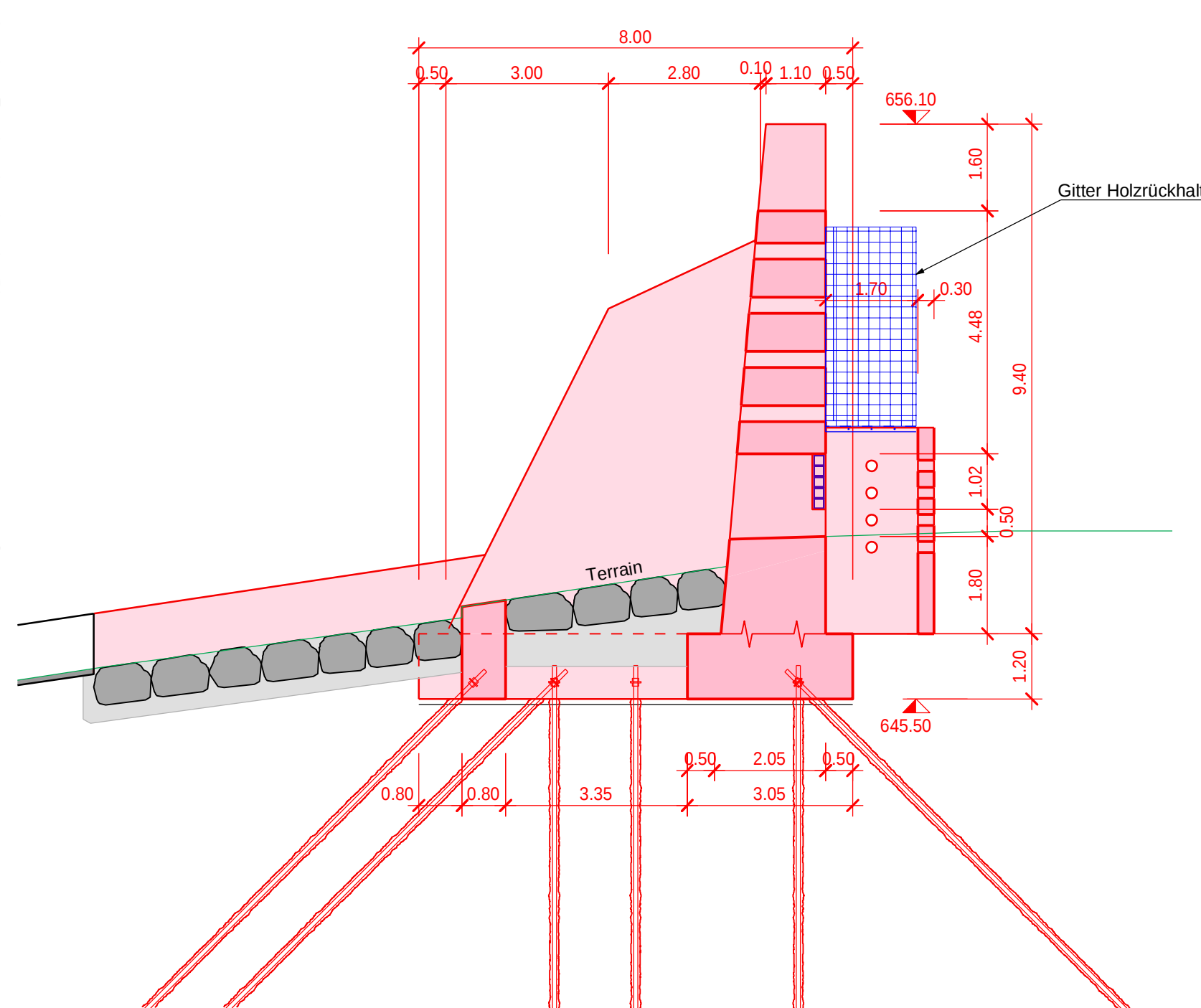
Schnitt B 1:100
