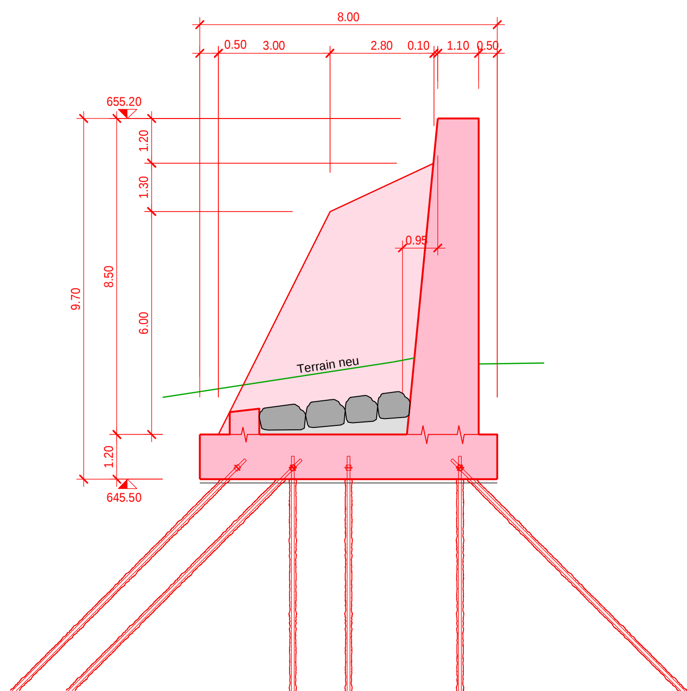
Schnitt A 1:100
