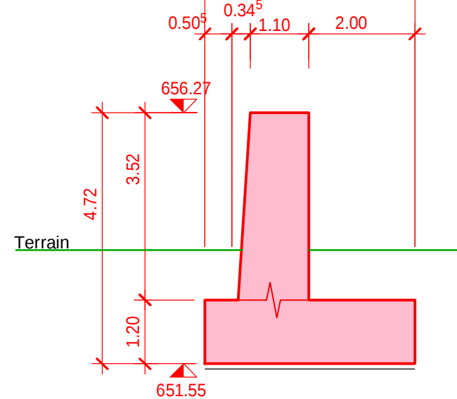
Schnitt G 1:100
